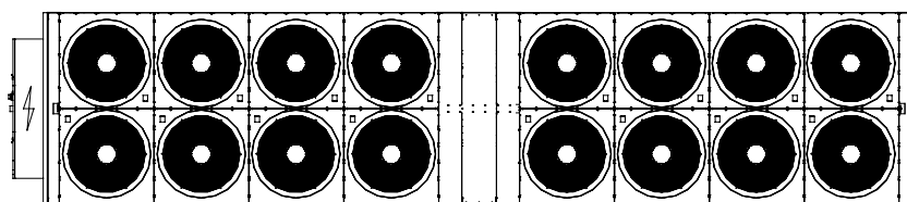
Схема расположения виброопор. 12 отверстий D14 для крепления виброопор
